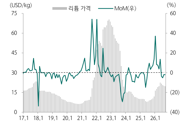
도표 127. 리튬 월별 평균 가격 추이
